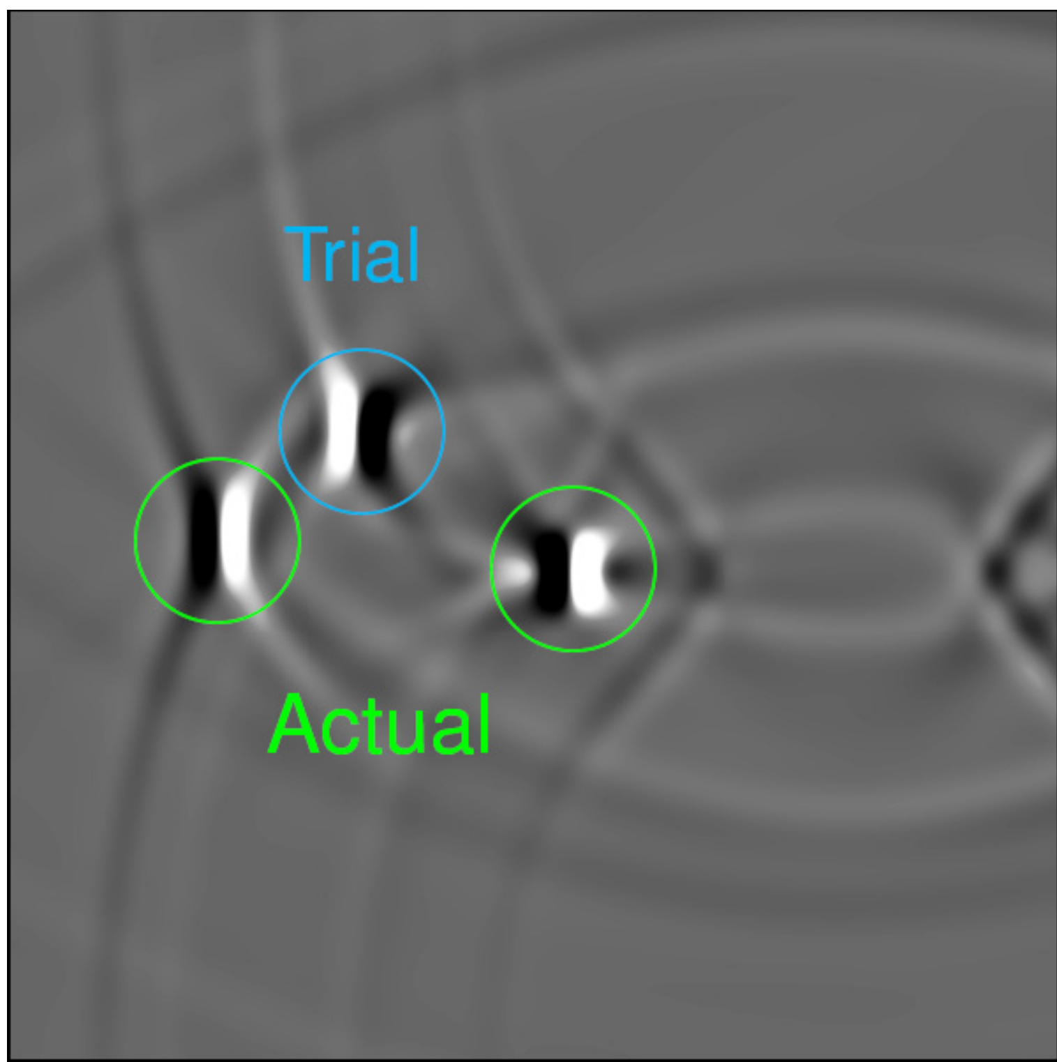
Adjoint wavefield
